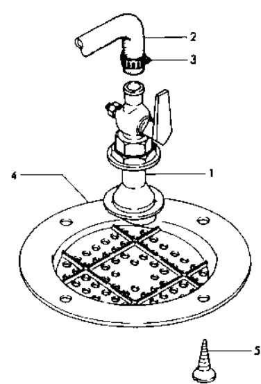
Fig. 38 キングストンコック KINGSTON COCK
