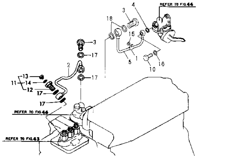
Fig.49 燃料パイプ FUEL PIPE
