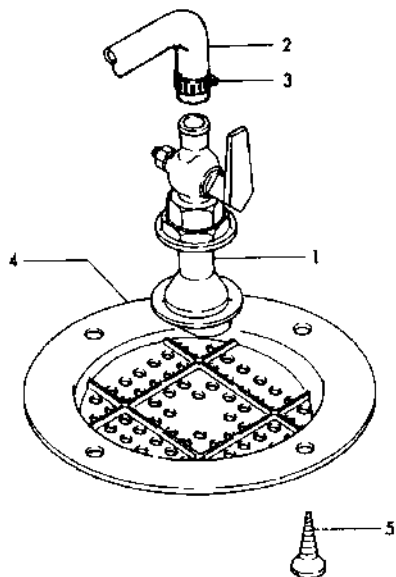
Fig. 76 キングストーンコック(オプション) KINGSTON COCK (OPTIONAL)
