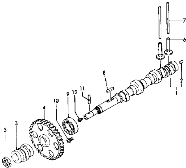
Fig.22 カムシャフト CAMSHAFT
