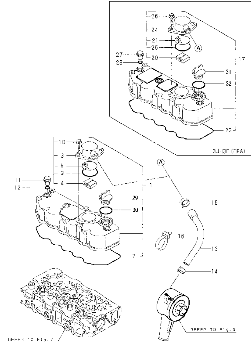
Fig.8 ボンネット&ブリーザ BONNET & BREATHER
