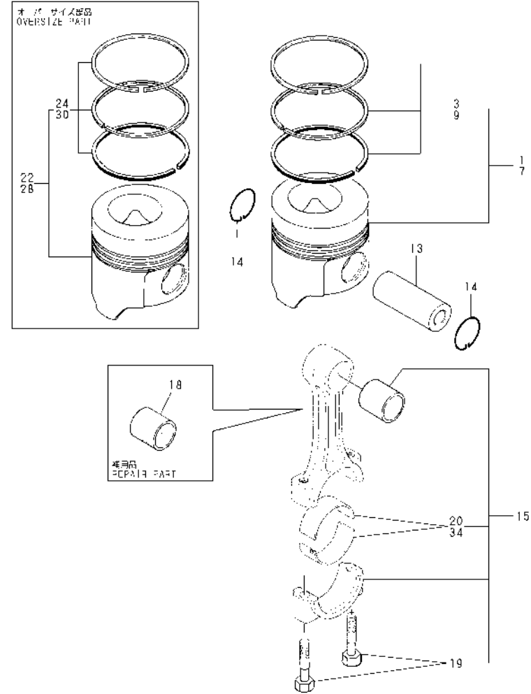
Fig. 13 ピストン&コネクティングロッド PISTON & CONNECTING ROD
