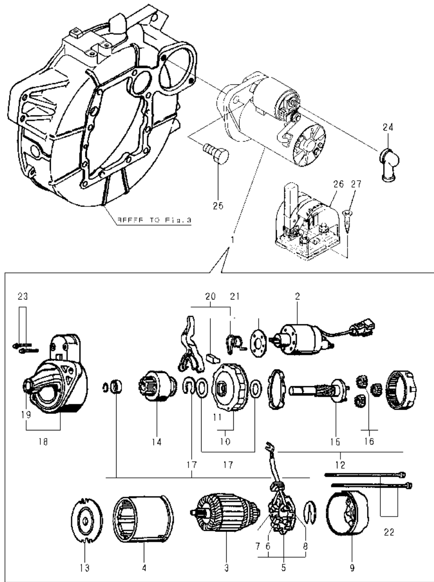
Fig.34 スターティングモータ STARTING MOTOR
