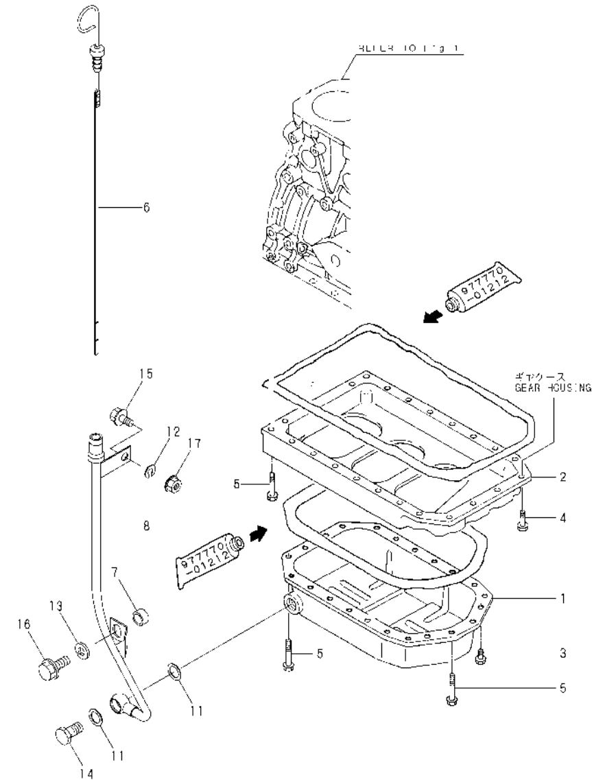
Fig.5 オイルパン LUB.OIL SUMP
