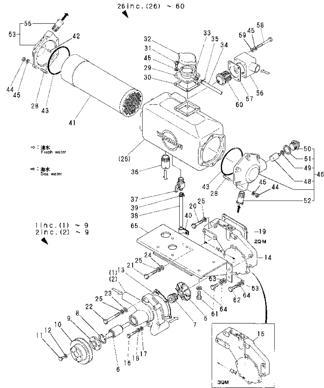
Fig.11. C.F.W.PUMP & C.F.W.COOLER
