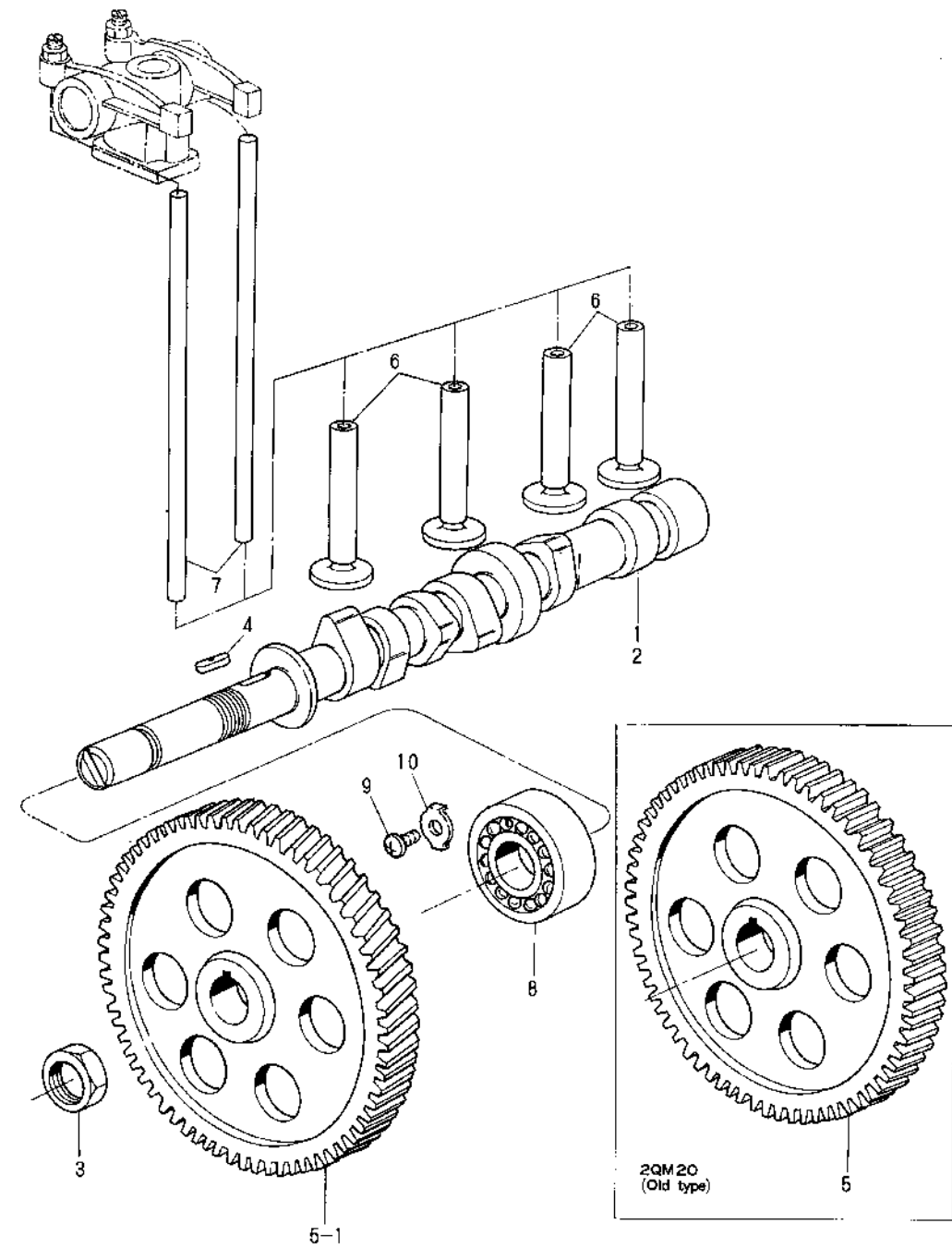
Fig.5. CAMSHAFT
