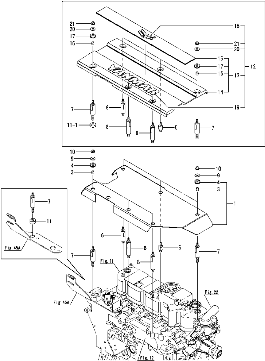
Fig.9. COVER(ENGINE)
