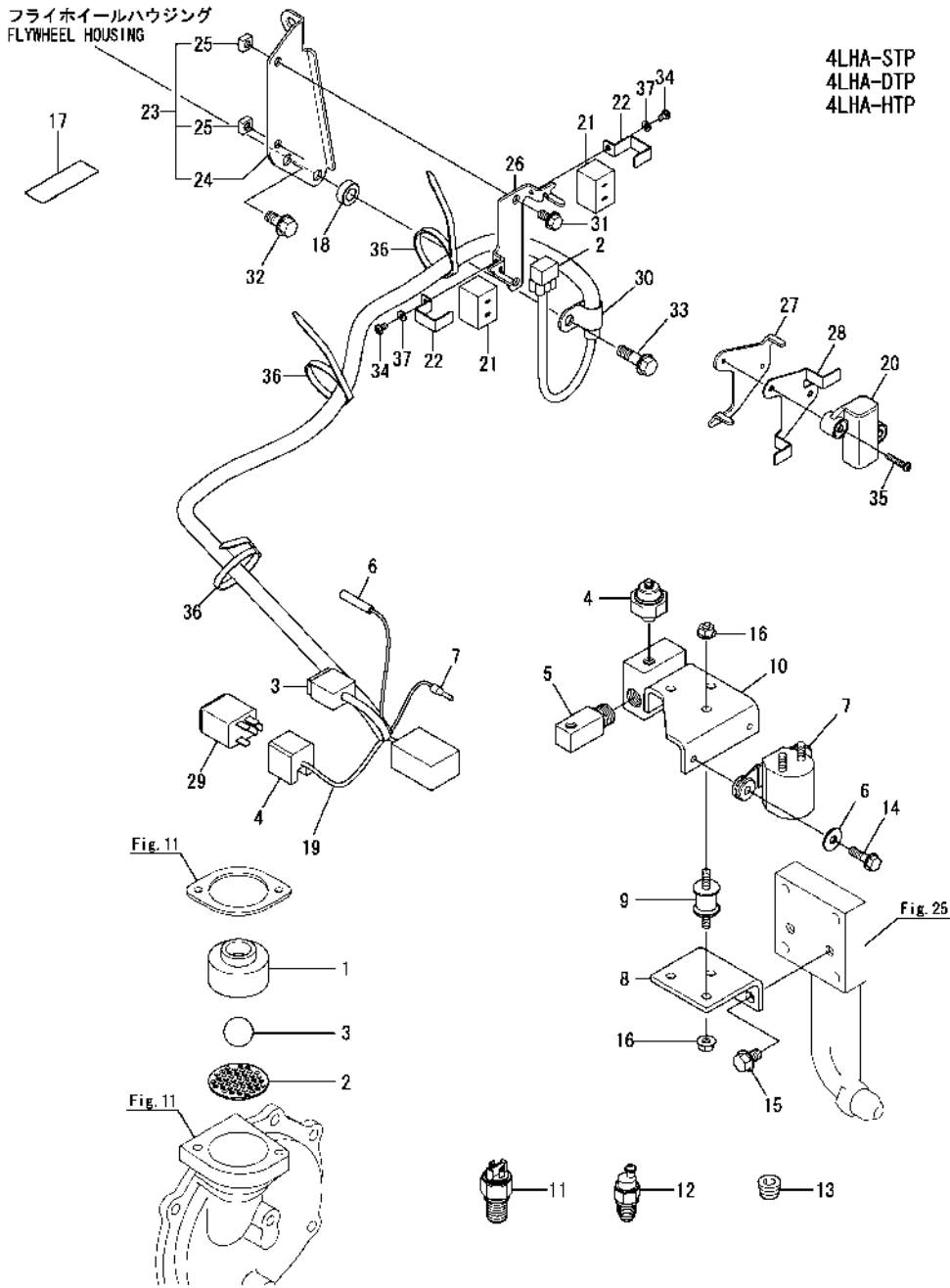
Fig.72. SOLAS SENSOR(OPTIONAL)
