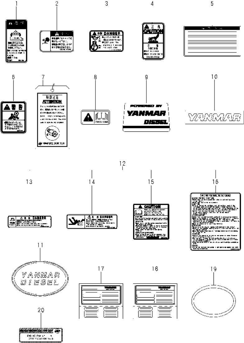
Fig.7 銘板 LABEL
