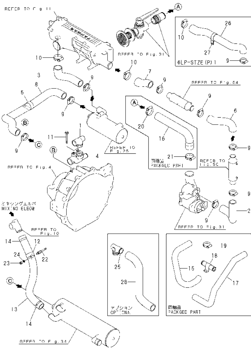
Fig. 38 冷却水パイプ (海水, 6LP-STZE (P) (1)) C. S. W. PIPE (6LP-STZE (P) (1))
