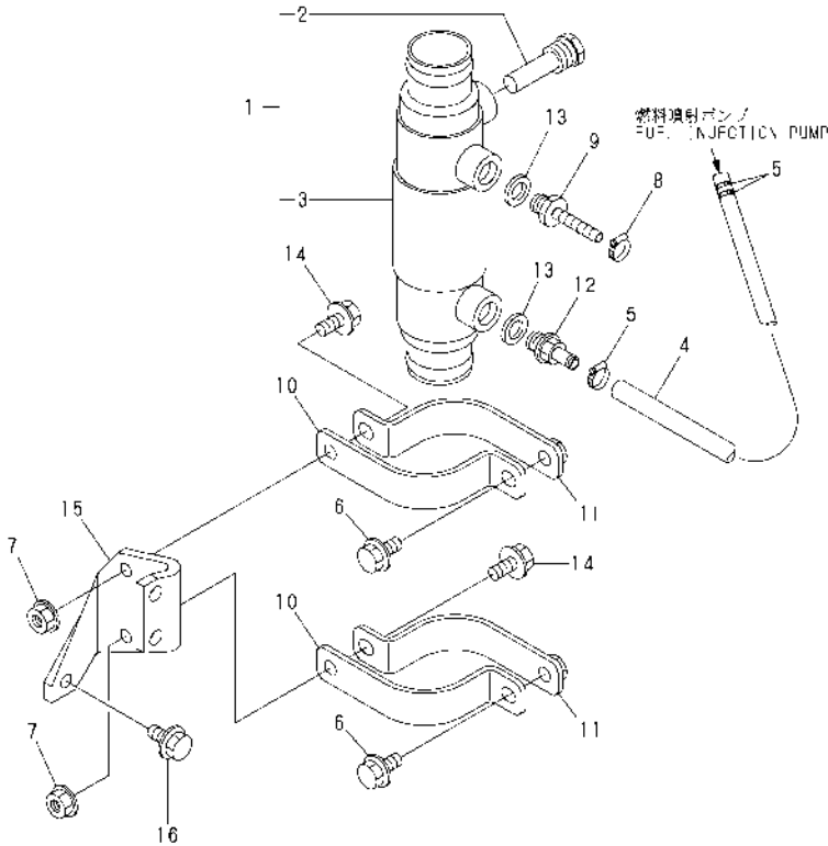
Fig.50 燃料クーラ FUEL COOLER
