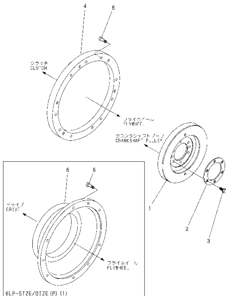
Fig. 22 ダンバ DAMPER
