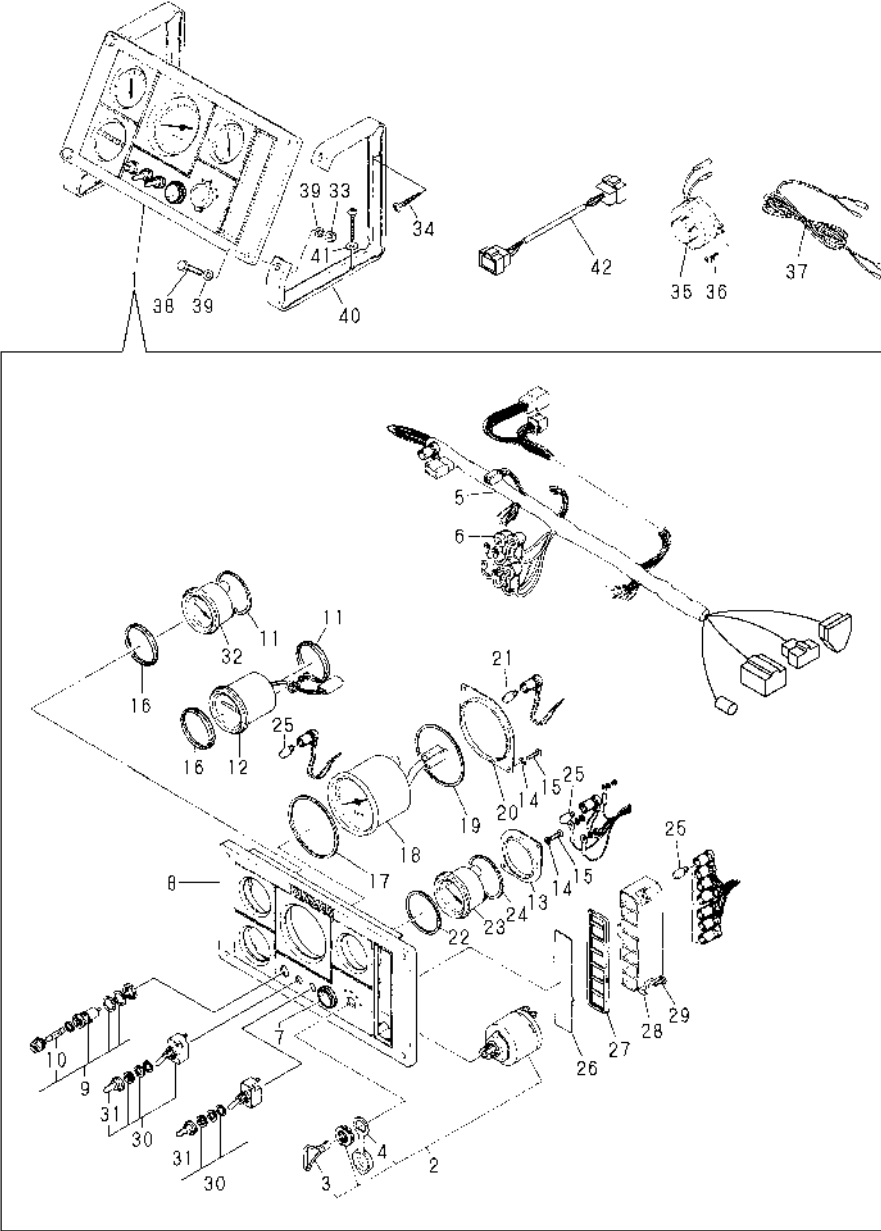
Fig.61. INSTRUMENT PANEL(C:4JH3-TE)
