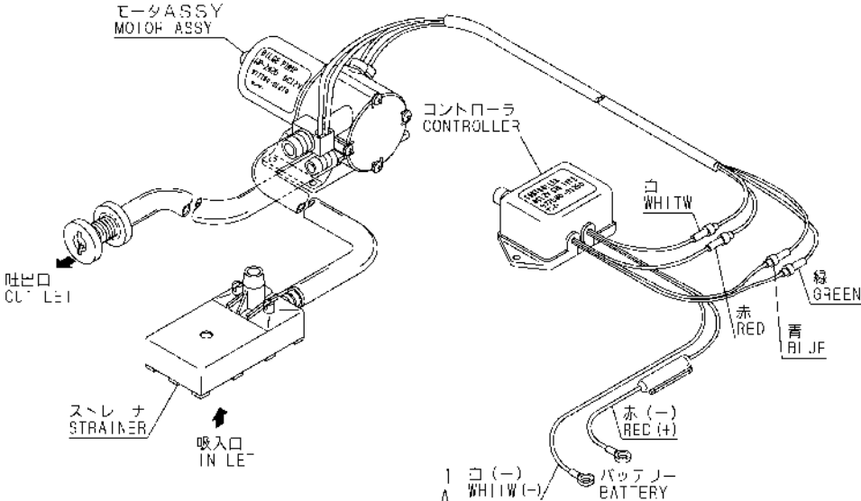
Fig.33. BILGE PUMP(STD)
