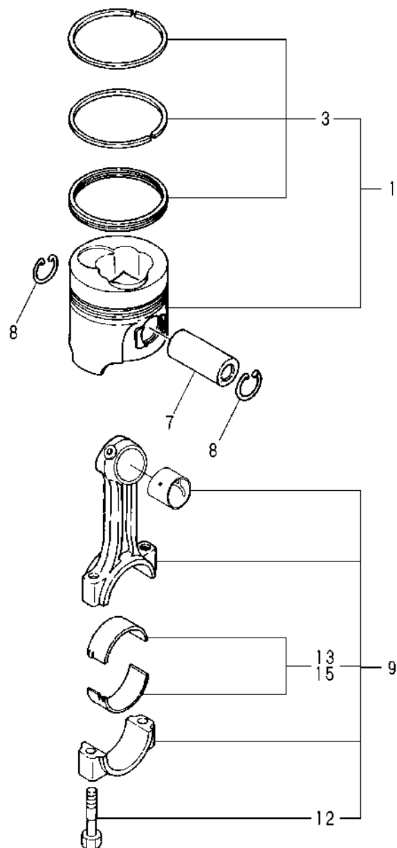
Fig.20. PISTON(4JH3-TE)
