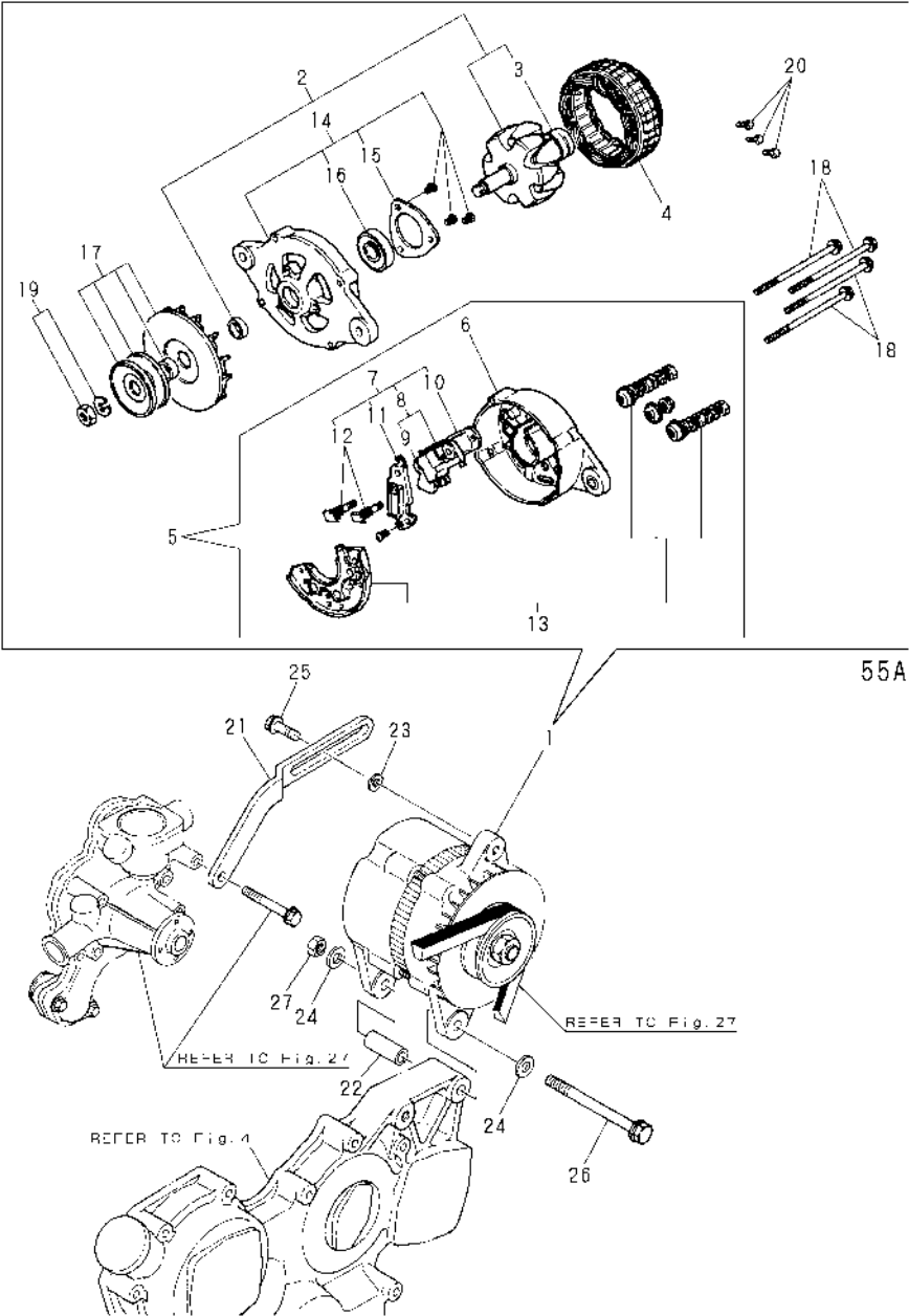
OCR10-M46701 4JH3E(CE/CE1)-TE(TCE) Fig.51. GENERATOR(4JH3-TE)
