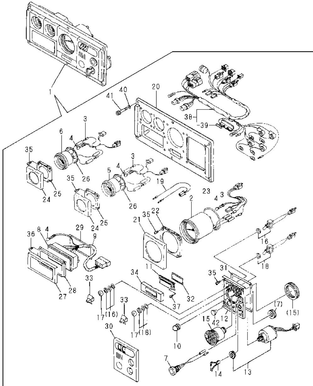
Fig.67. PANEL(C:NEW TYPE:PREVOUS)
