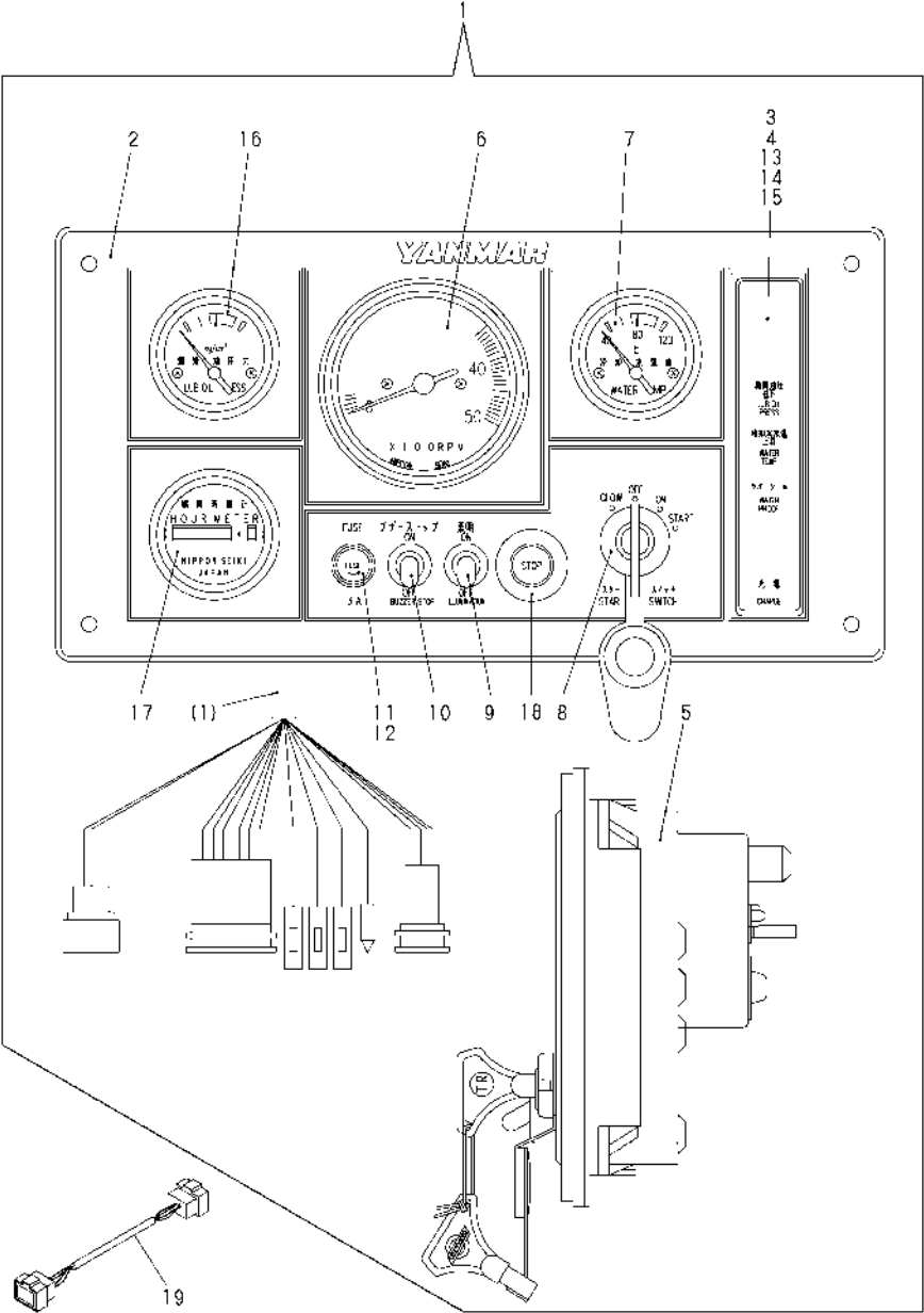
OCR10-M46701 4JH3E(CE/CE1)-TE(TCE) Fig.59. INSTRUMENT PANEL(C:4JH3E)
