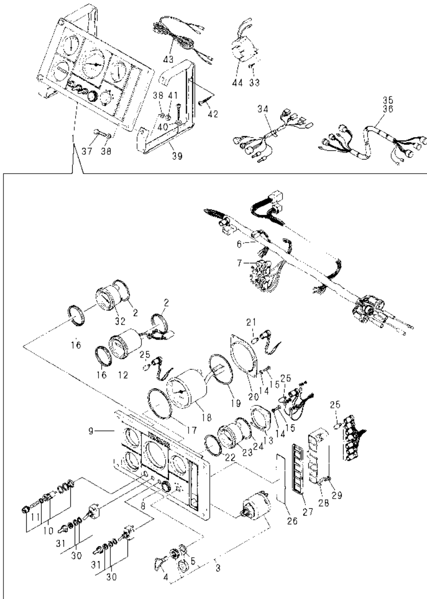
Fig.60. INSTRUMENT PANEL(C:4JH3-TE)
