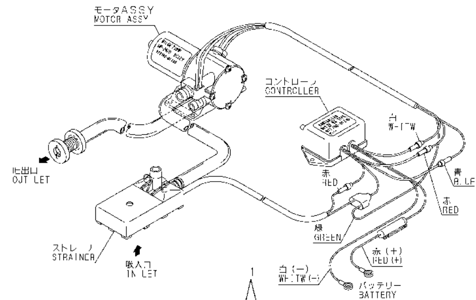
Fig.34. BILGE PUMP(DX)
