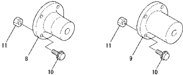
ストレートカップリング STRAIGHT COUPLING
